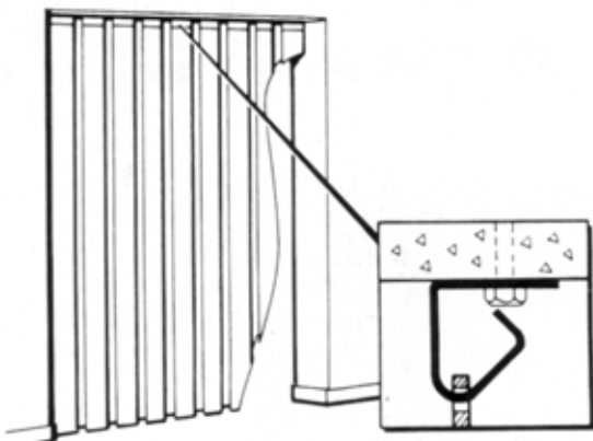
TYPE 1 FOR MONTAGE I DØRÅBNING
