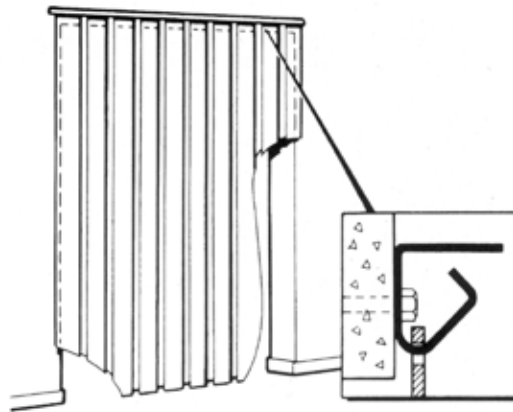
TYPE 2 FOR MONTAGE FORAN DØRÅBNING
